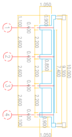
SECCION TRANSVERSAL CORTE (A-A) ESCALA 1_125
