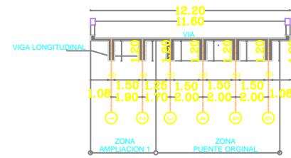
CORTE TRANSVERSAL A-A' ESC:1/200
