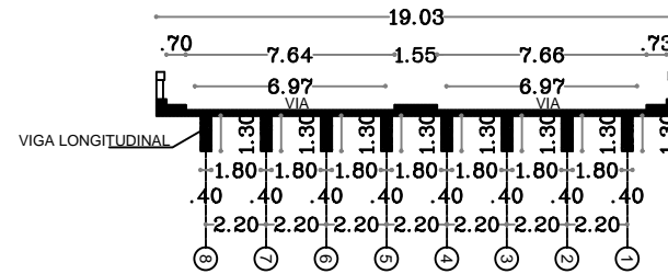
CORTE TRANSVERSAL A-A' ESC:1_200
