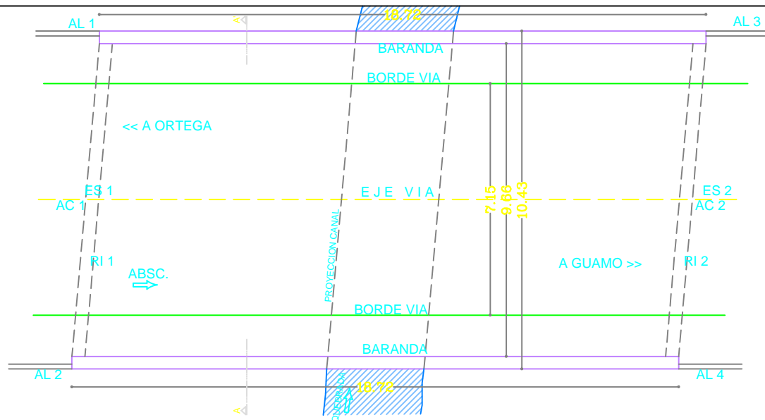
PLANTA GENERAL ESC:1_100
