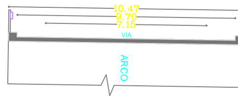
CORTE TRANSVERSAL A-A' ESC:1_100
