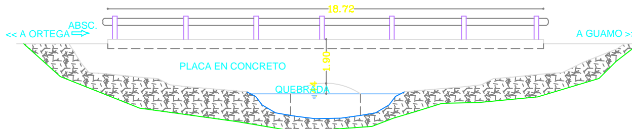
PERFIL LONGITUDINAL ESC:1_100
