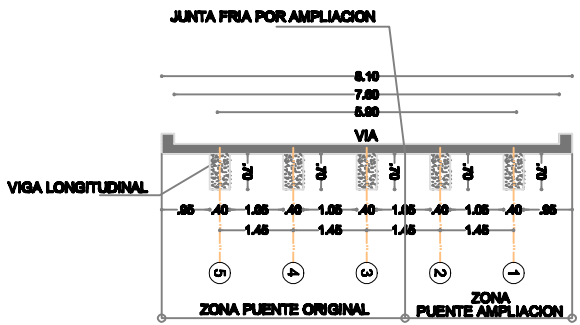
CORTE TRANSVERSAL A-A' ESC:1_100
