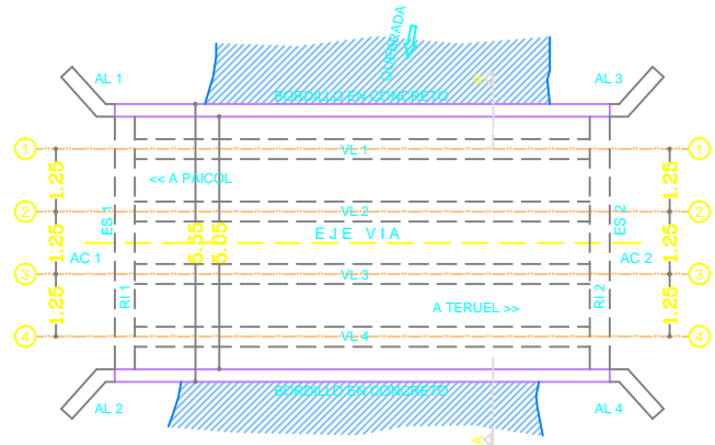
PLANTA GENERAL ESC:1_100
