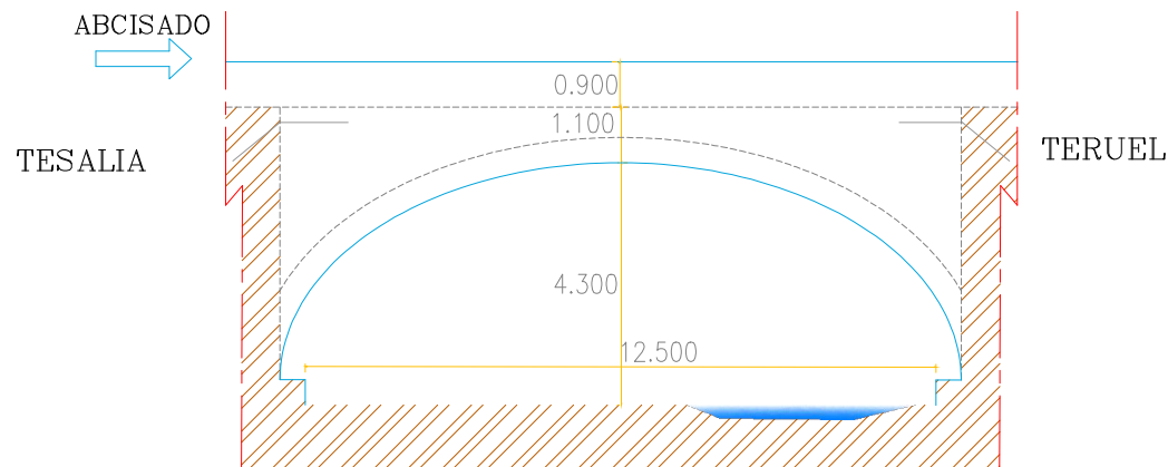
SECCION LONGITUDINAL ESCALA 1_100
