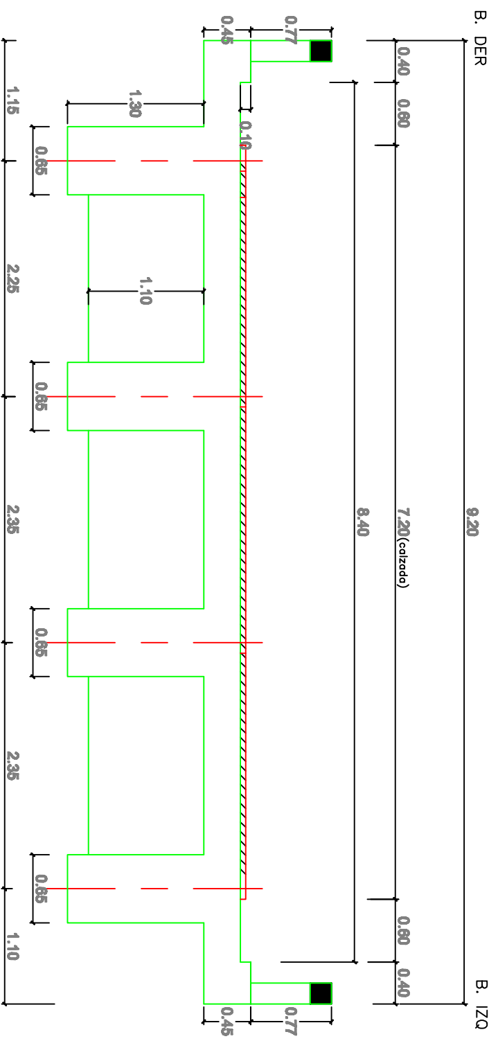
SECCION TRANSVERSAL CORTE A - A' ESCALA 1 : 50
