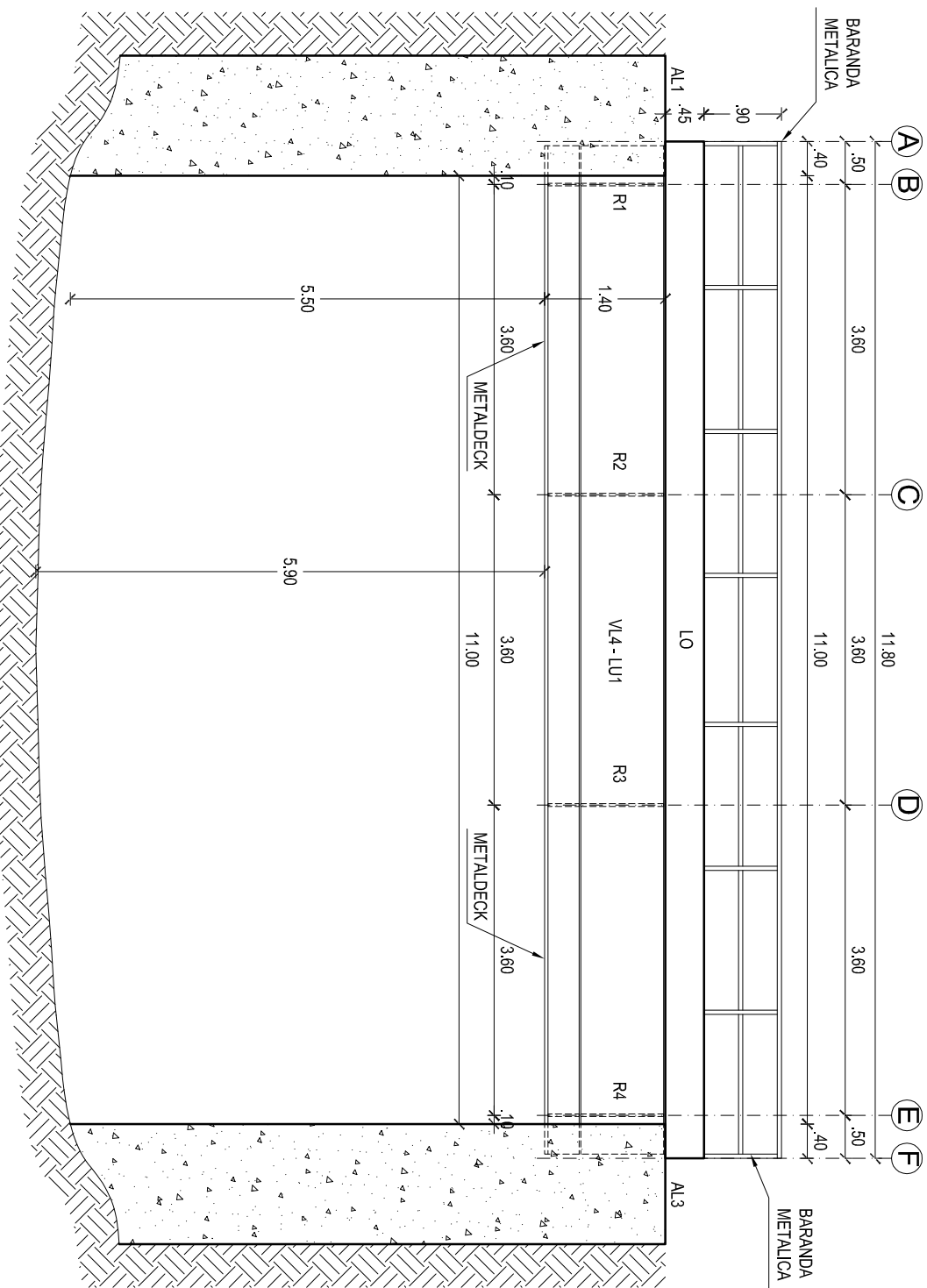
SECCIÓN LONGITUDINAL ESC 1:75
