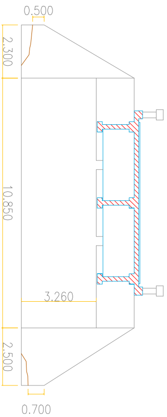
CORTE (B-B') ES2 ESCALA 1_100
