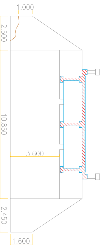
CORTE (A-A') ES1 ESCALA 1_100
