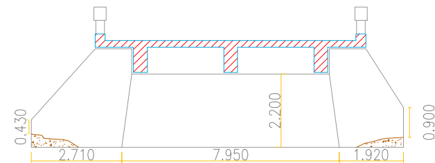
CORTE (B-B') ES2
