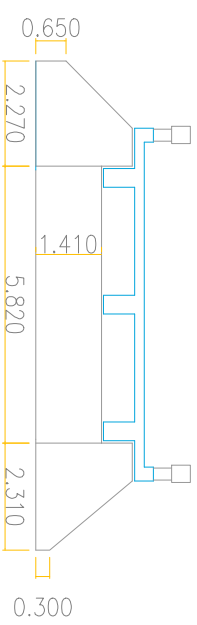
CORTE (B-B') ES2
