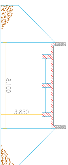
VISTA ESI (CORTE A-A')
