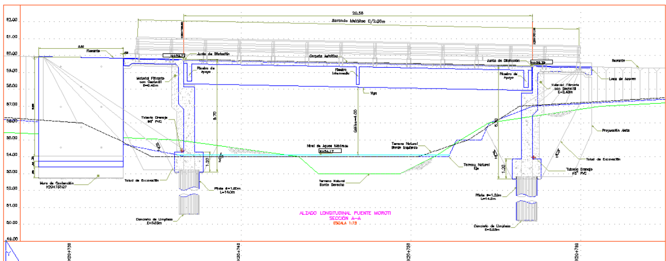
Perfil Longitudinal Puente
