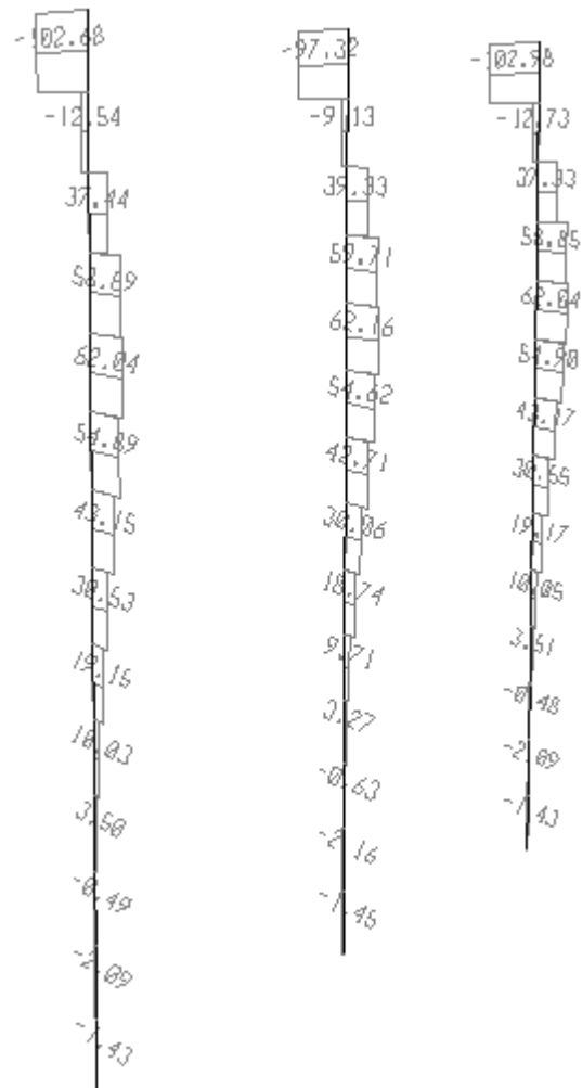
Cortantes Últimos Sentido al Tráfico (Ton)
