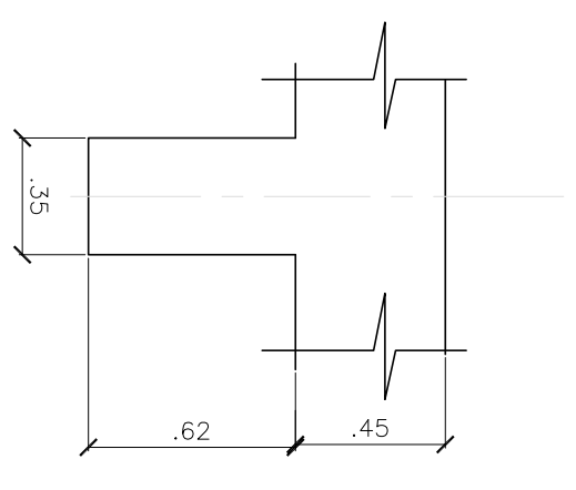
SECCION TRANSVERSAL VIGA LONGITUDINAL
