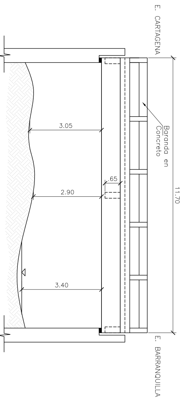
SECCION LONGITUDINAL (B-B')
