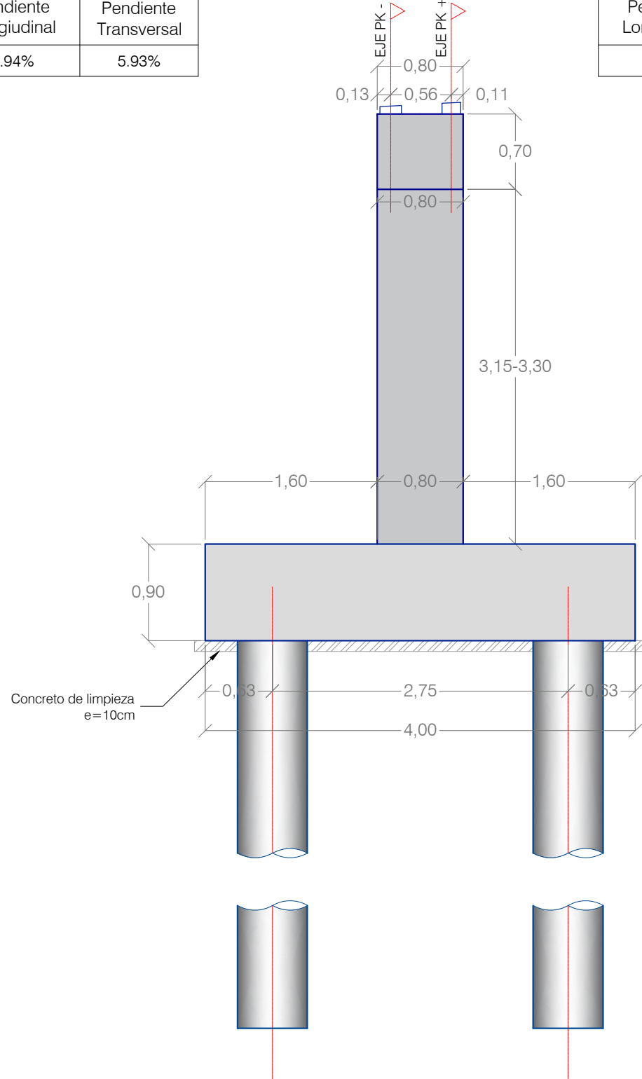
PÓRTICO 11 PERFIL
