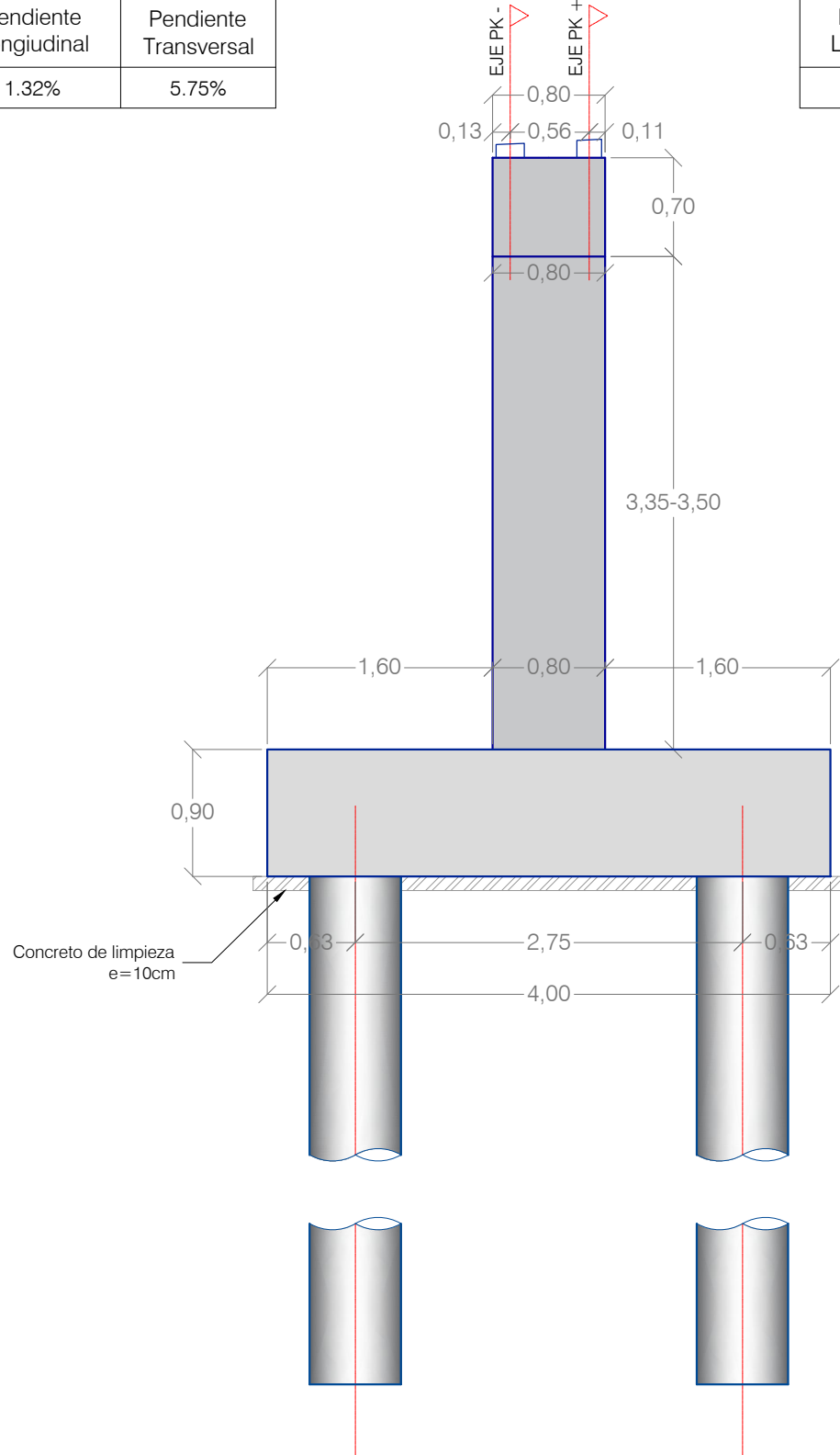
PÓRTICO 10 PERFIL
