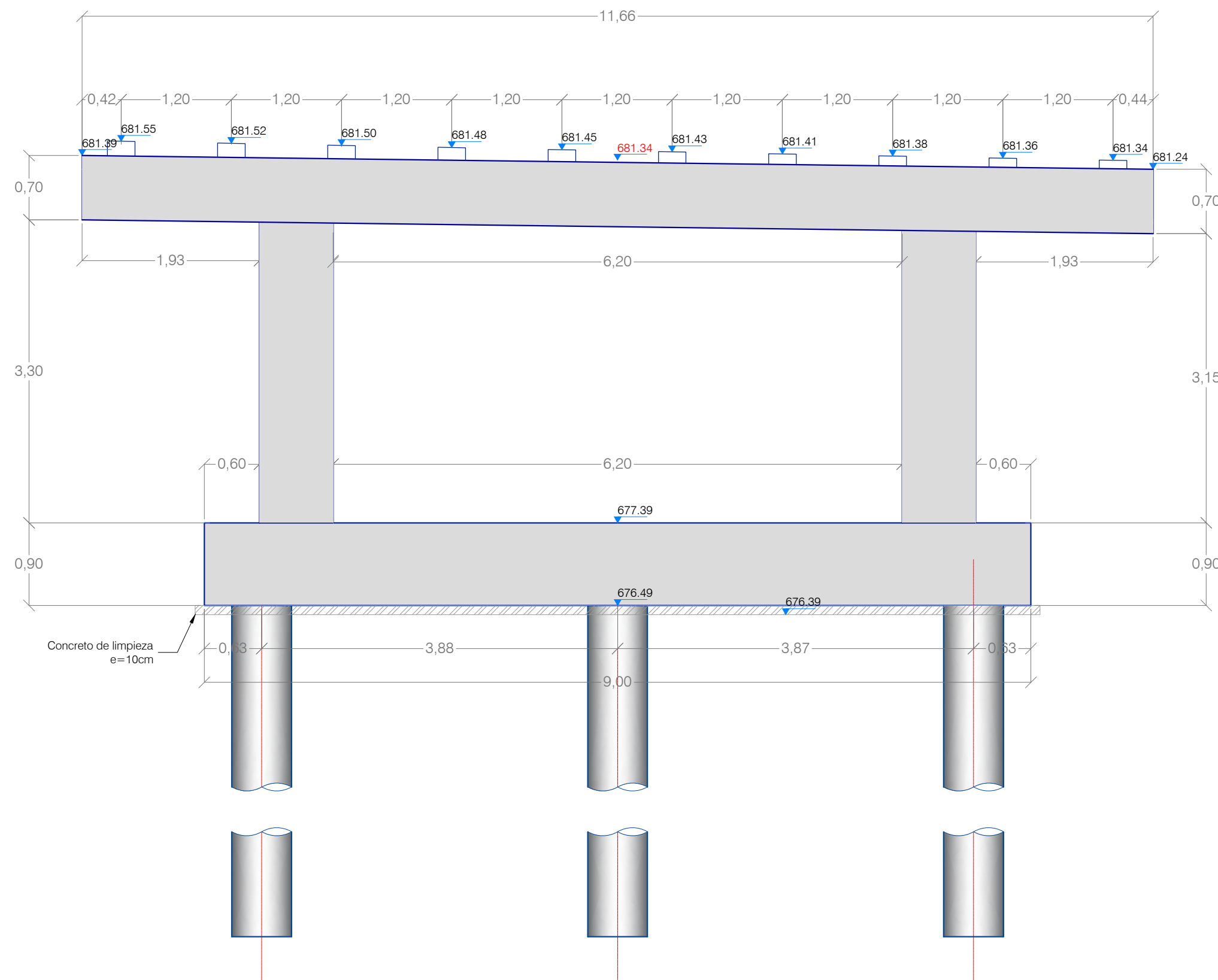
PÓRTICO 11 PK -
