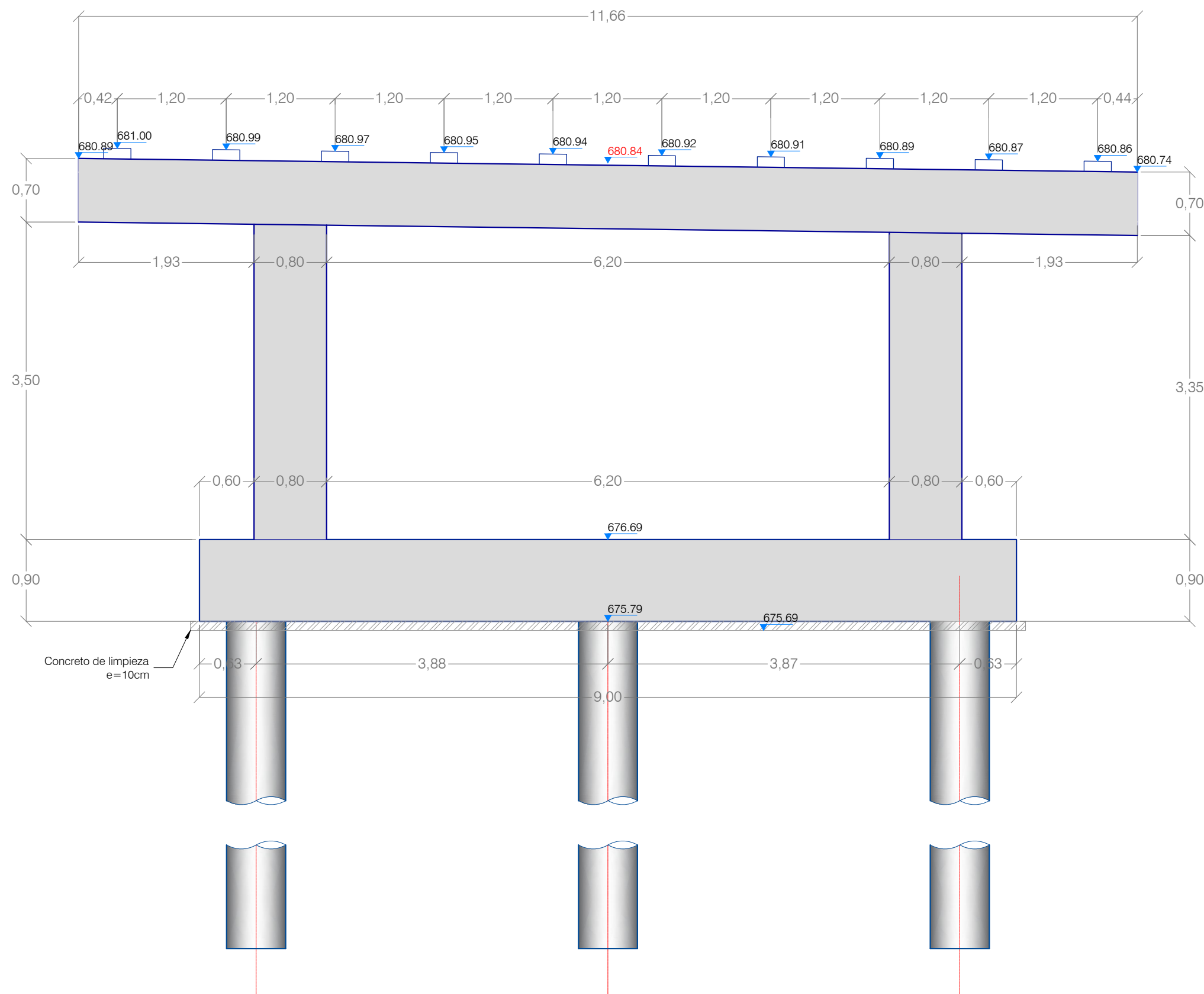
PÓRTICO 10 PK -
