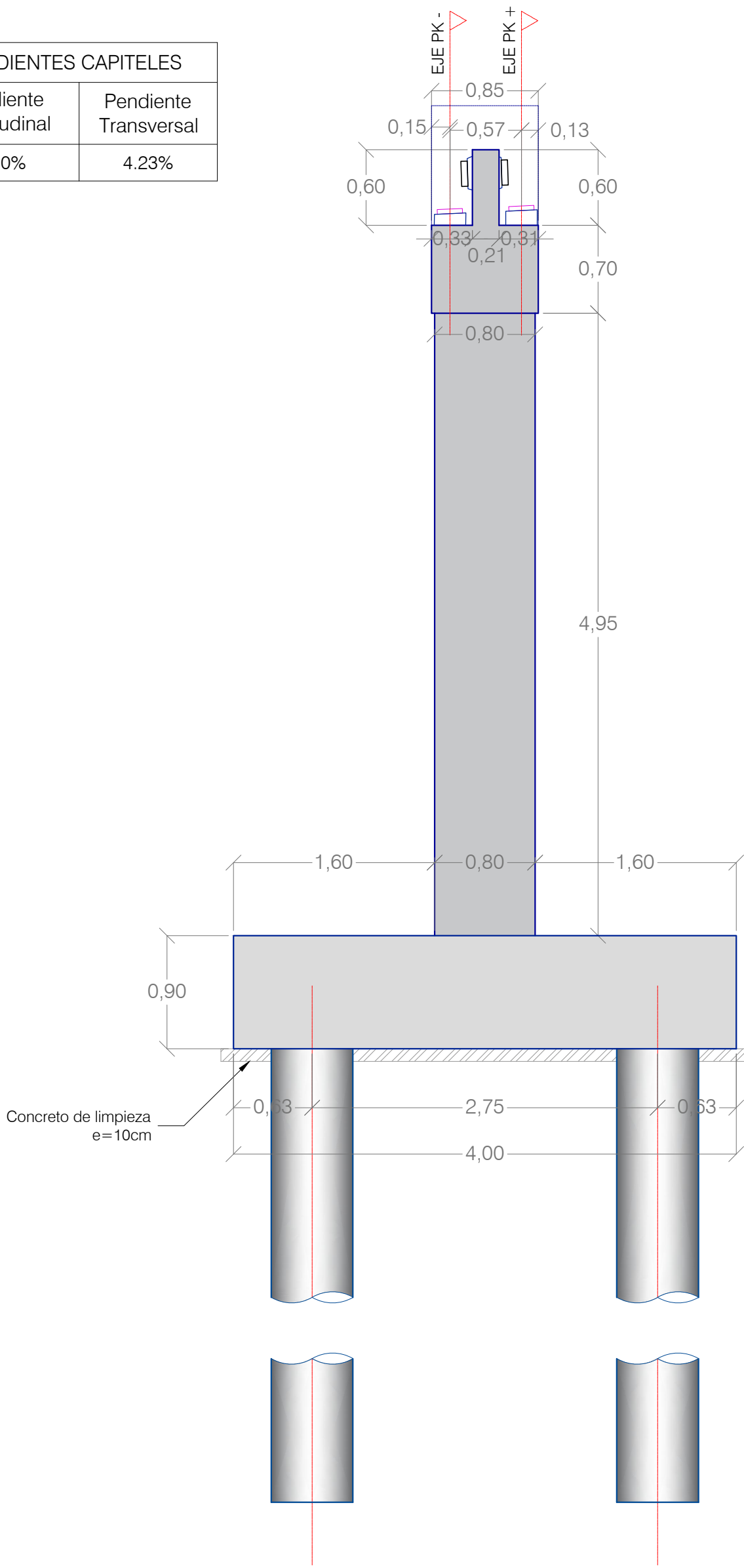
PÓRTICO 6 PERFIL
