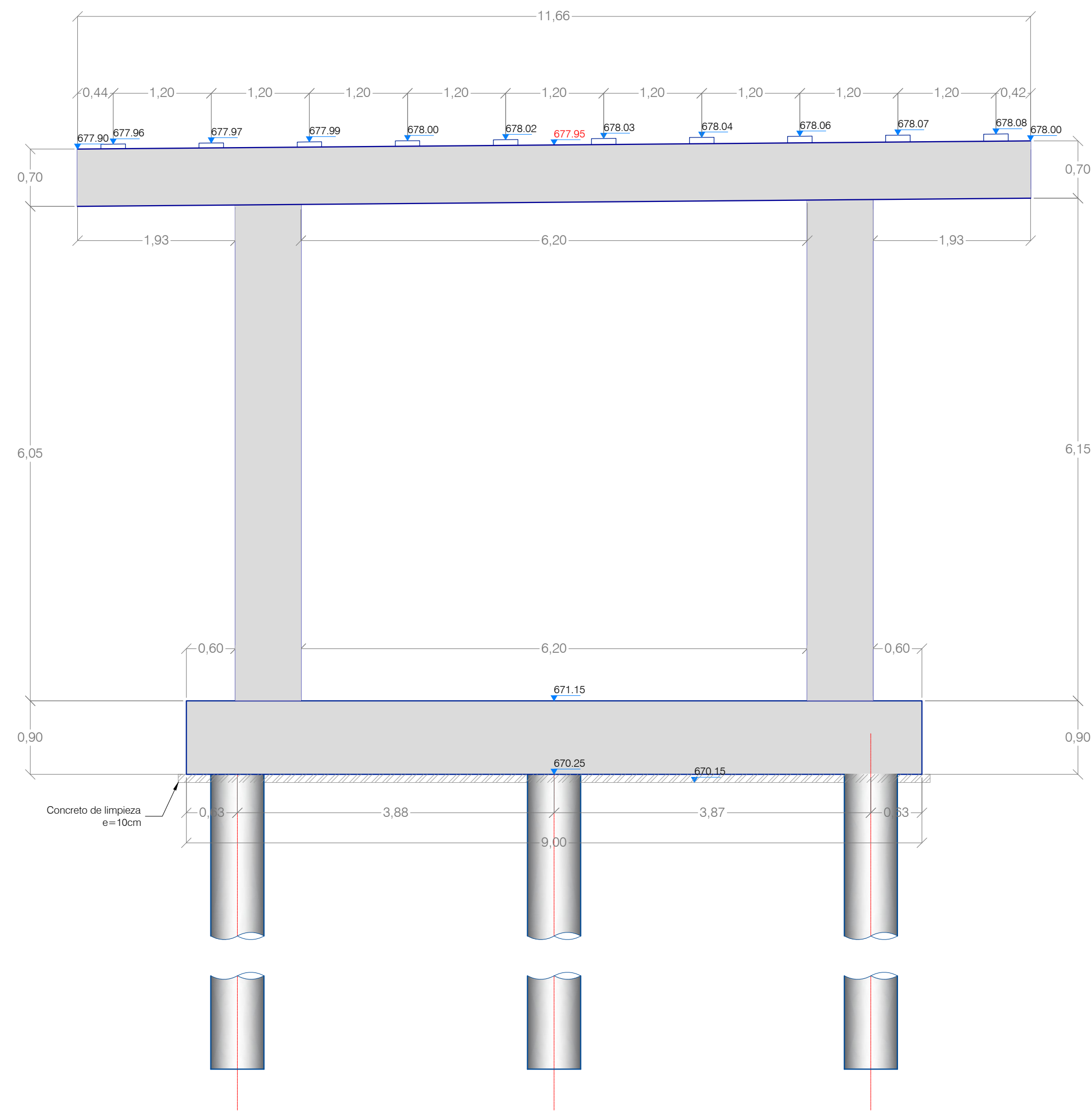
PÓRTICO 4. PK -
