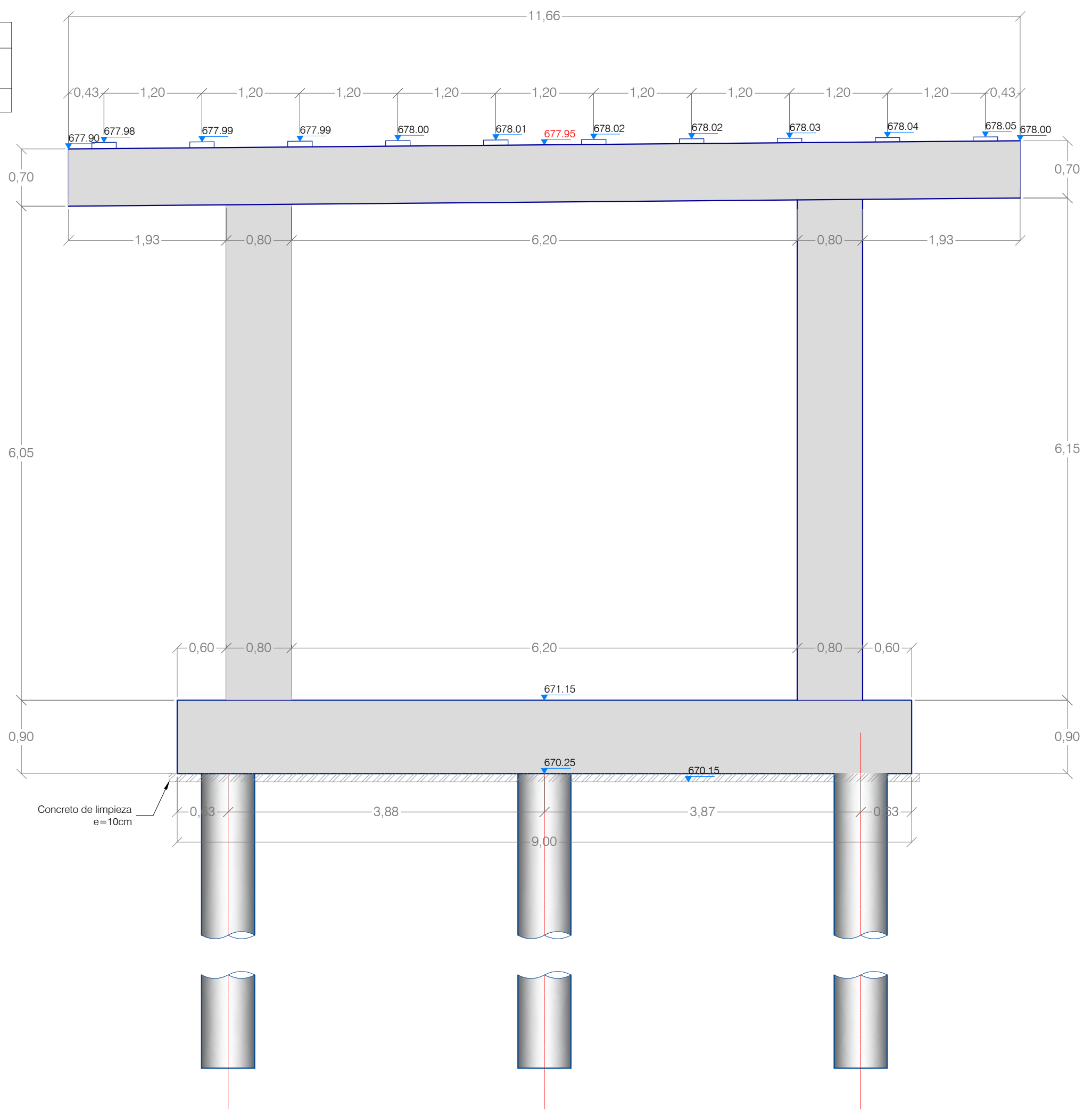
PÓRTICO 4. PK +
