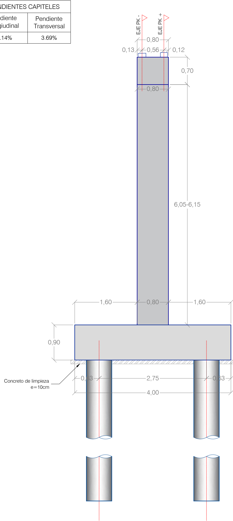
PÓRTICO 4 PERFIL
