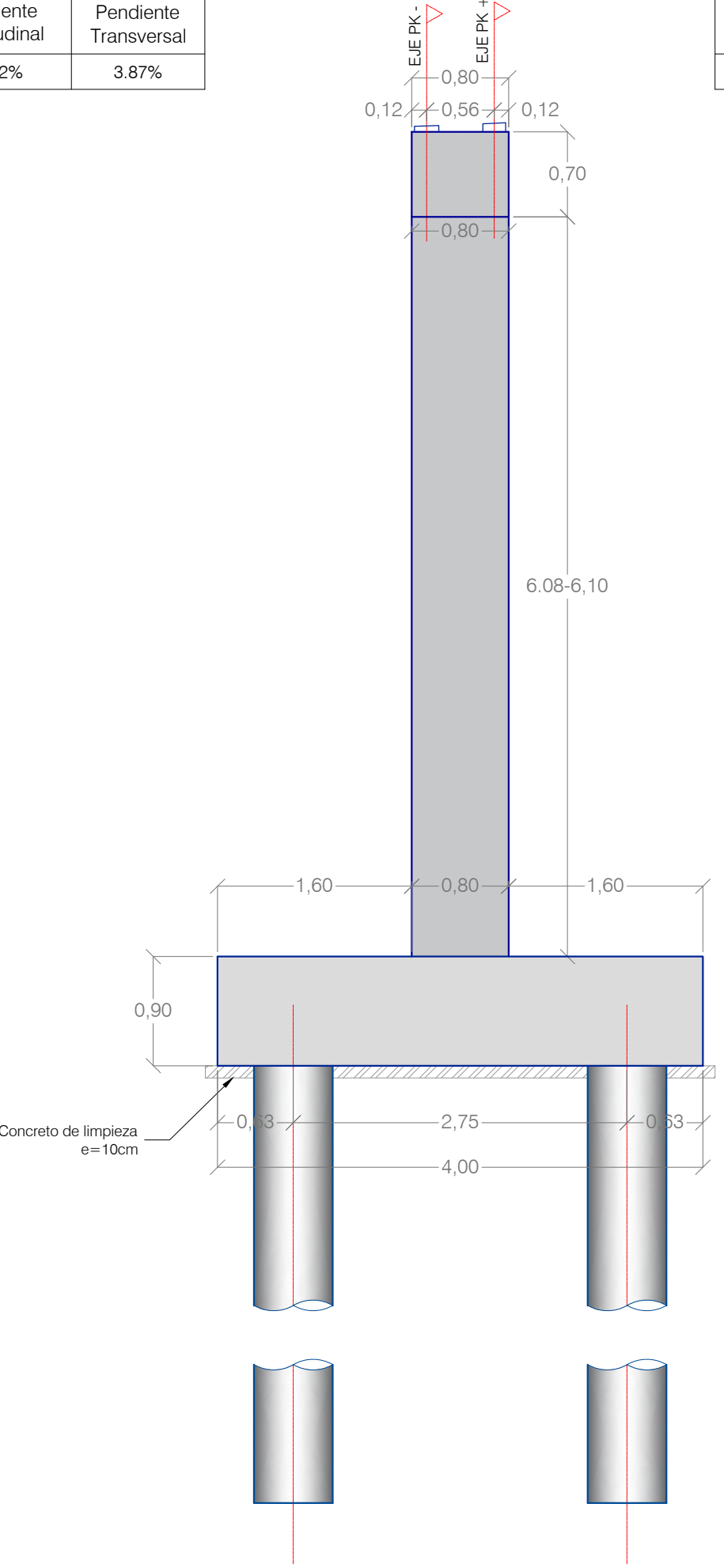
PÓRTICO 4 PERFIL
