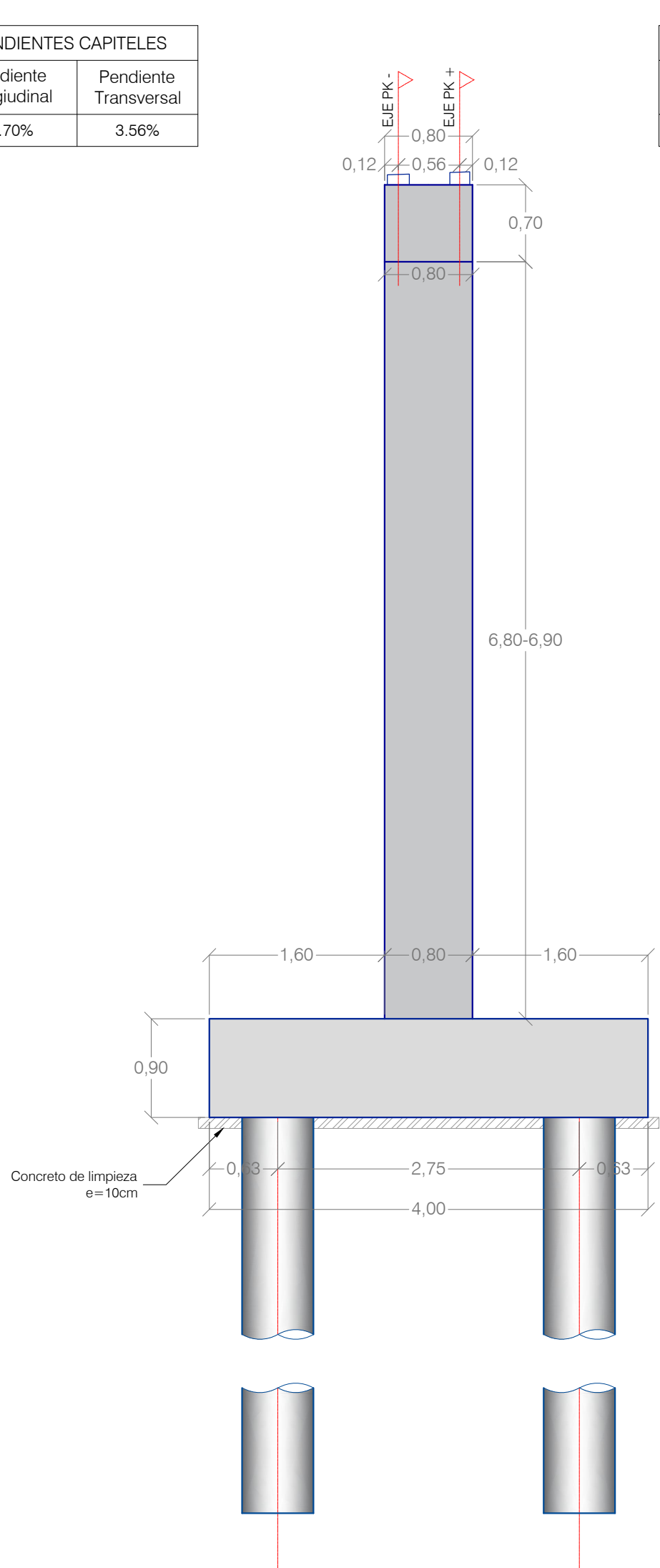
PÓRTICO 2 PERFIL
