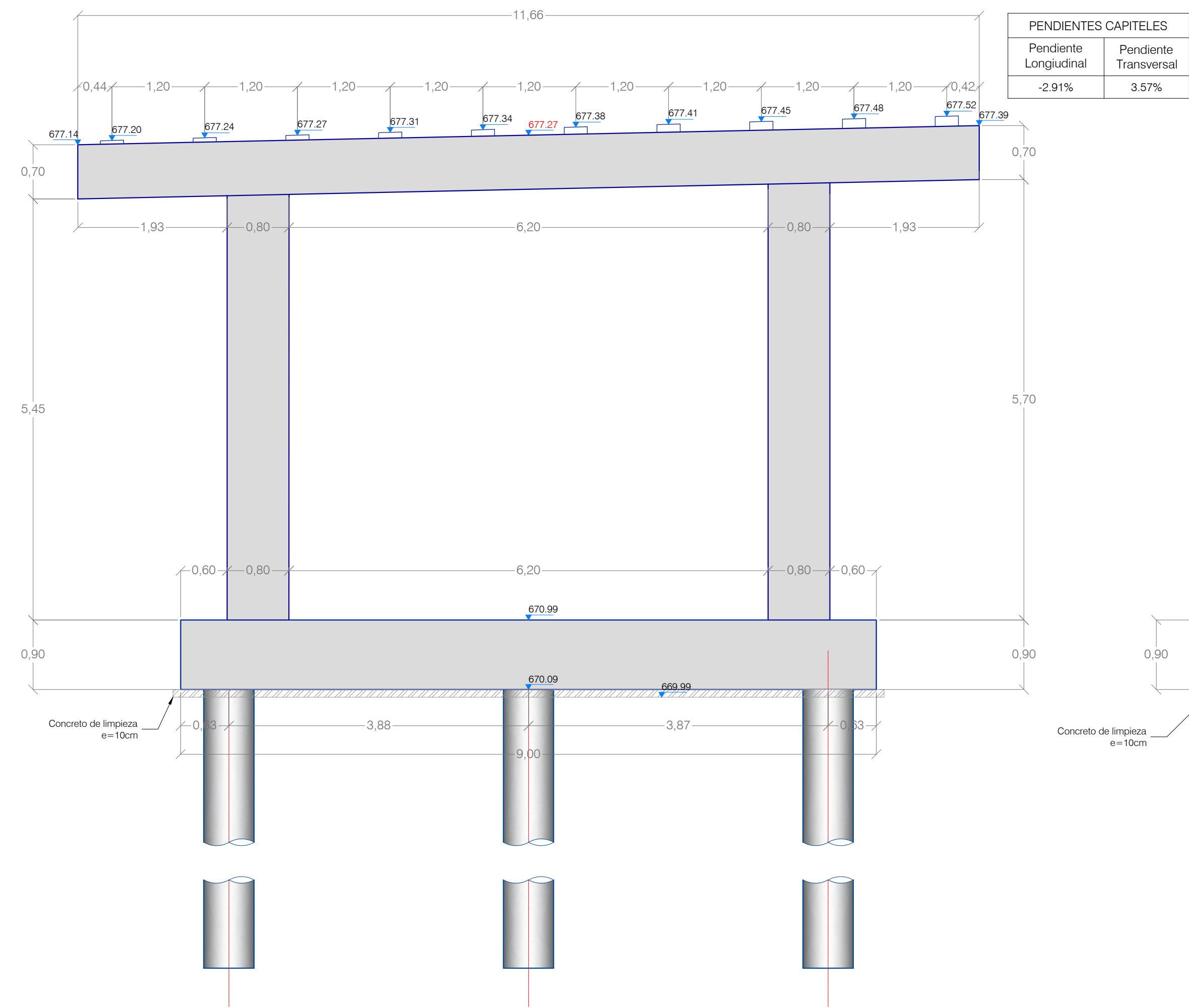
PÓRTICO 2. PK -
