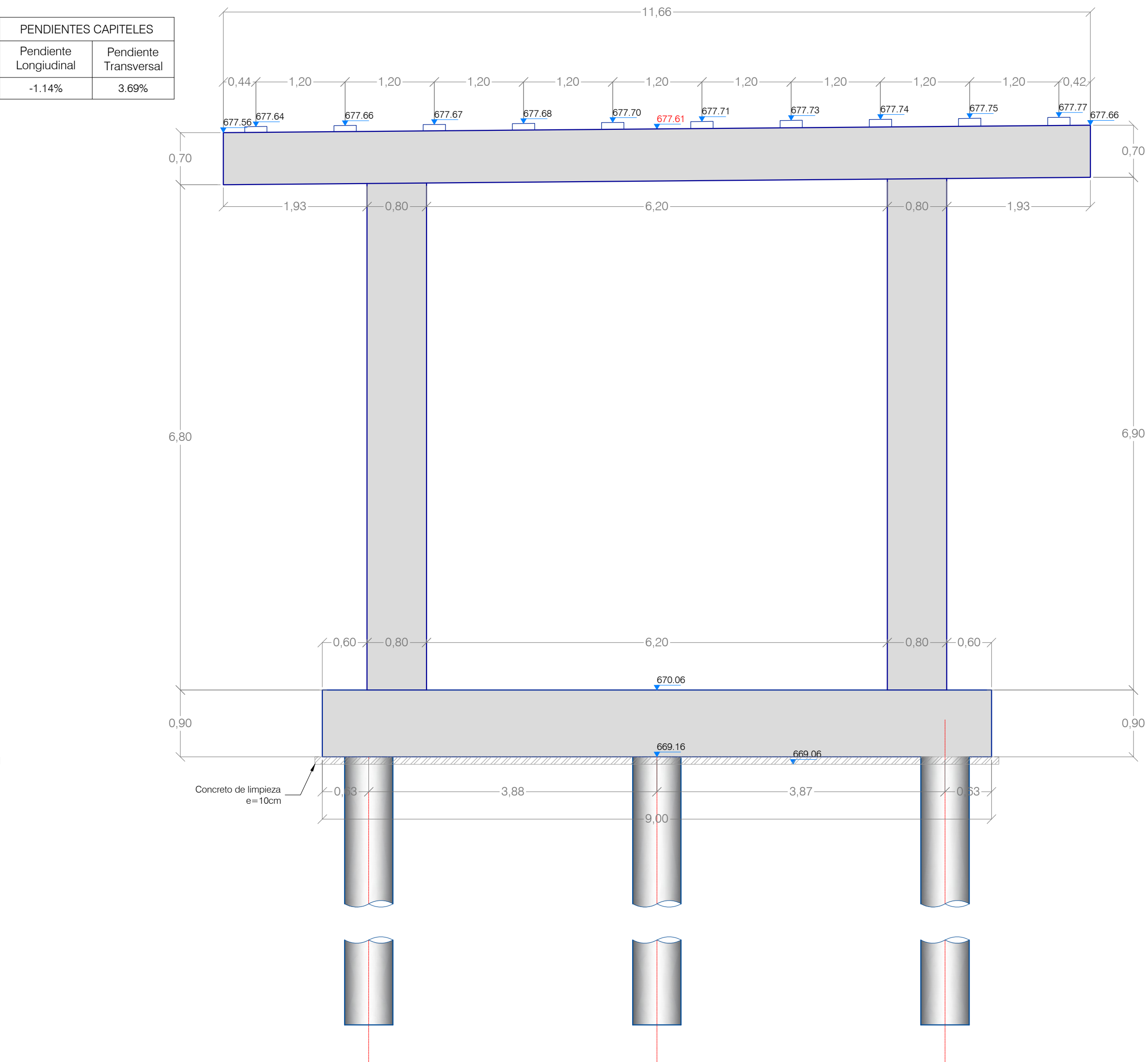
PÓRTICO 2. PK +
