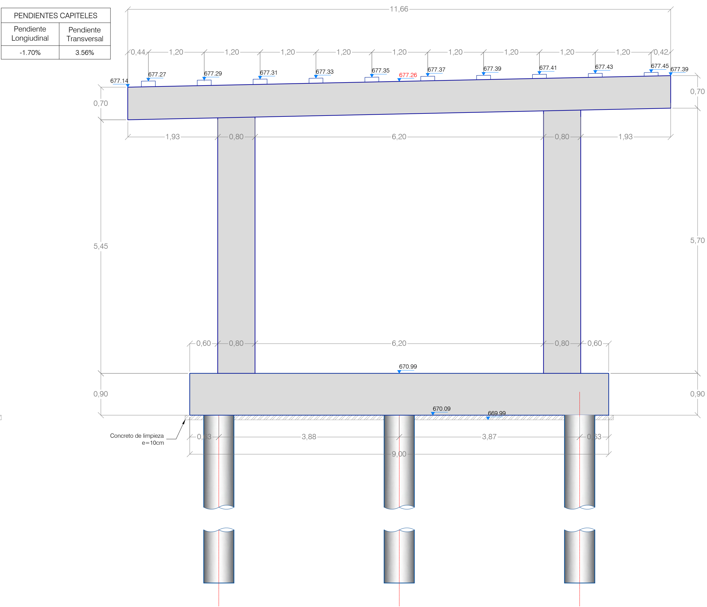
PÓRTICO 2. PK +
