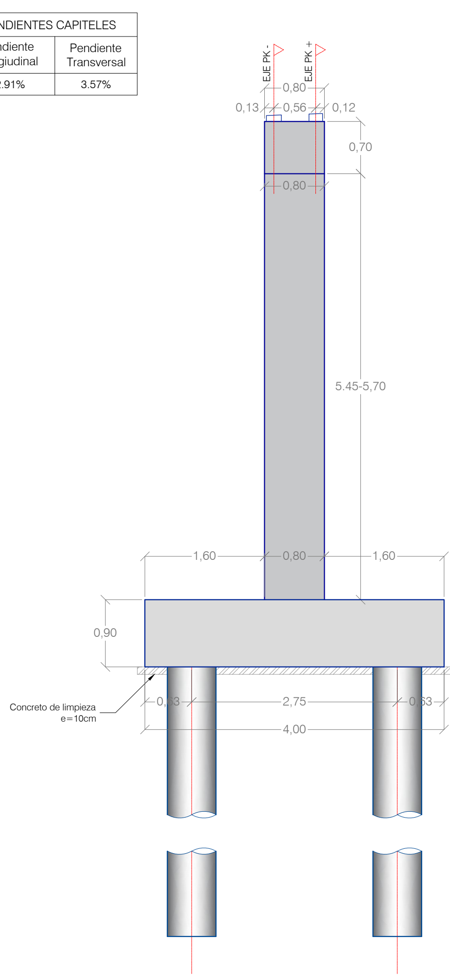
PÓRTICO 2 PERFIL
