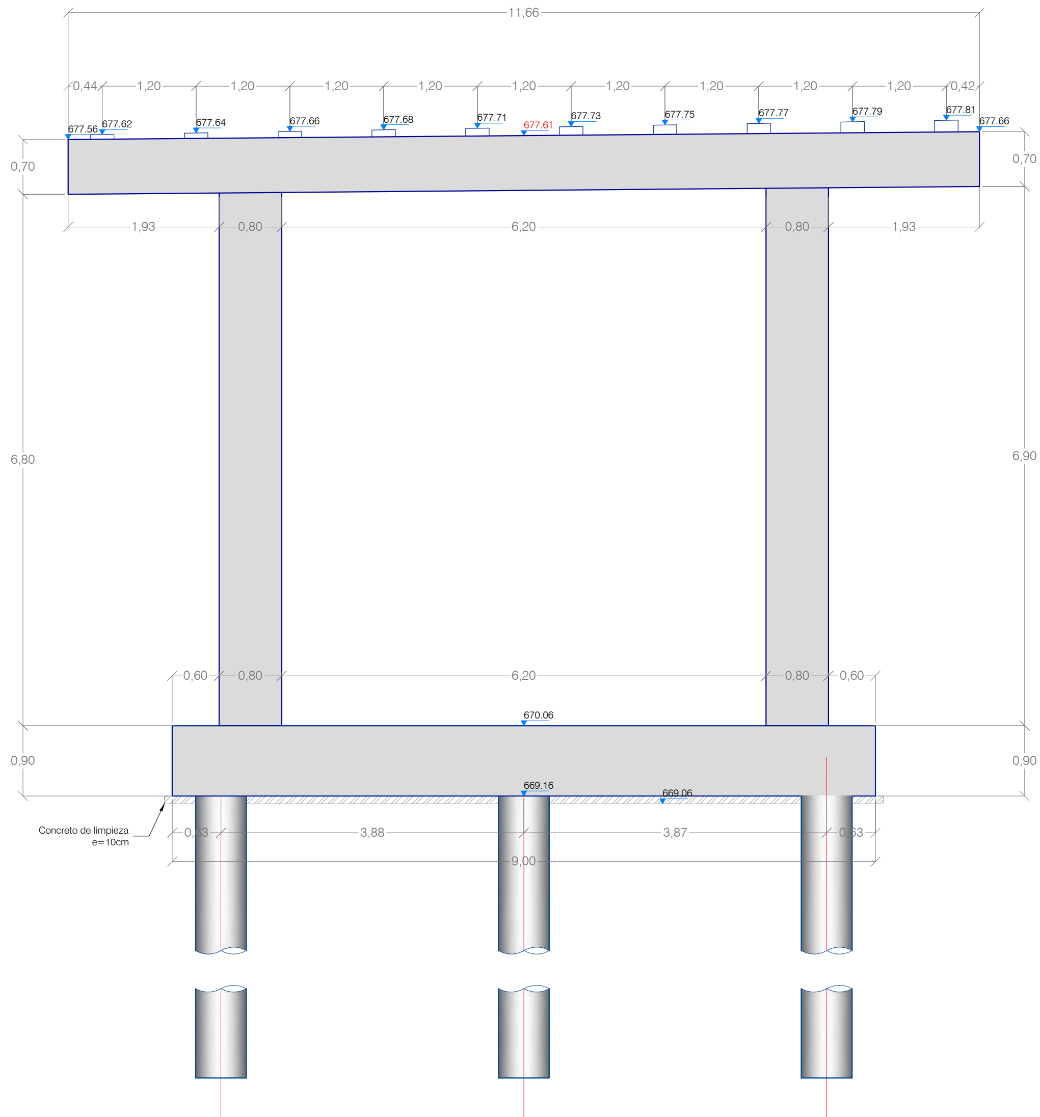
PÓRTICO 2. PK -
