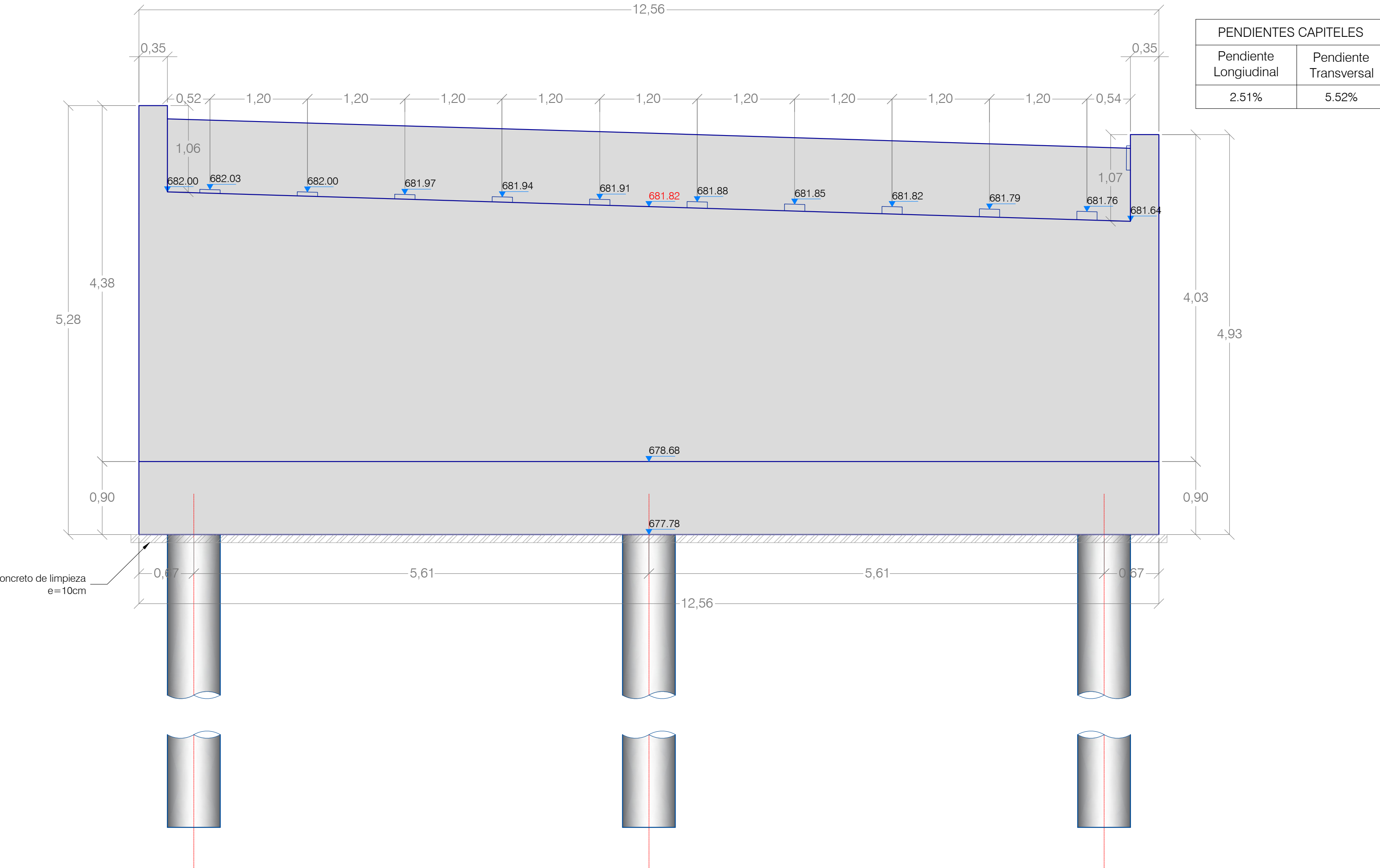
ESTRIBO 2 ALZADO
