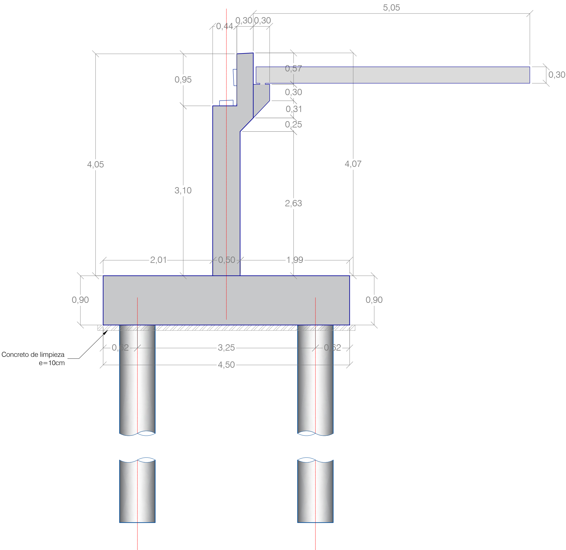
ESTRIBO 1 PERFIL
