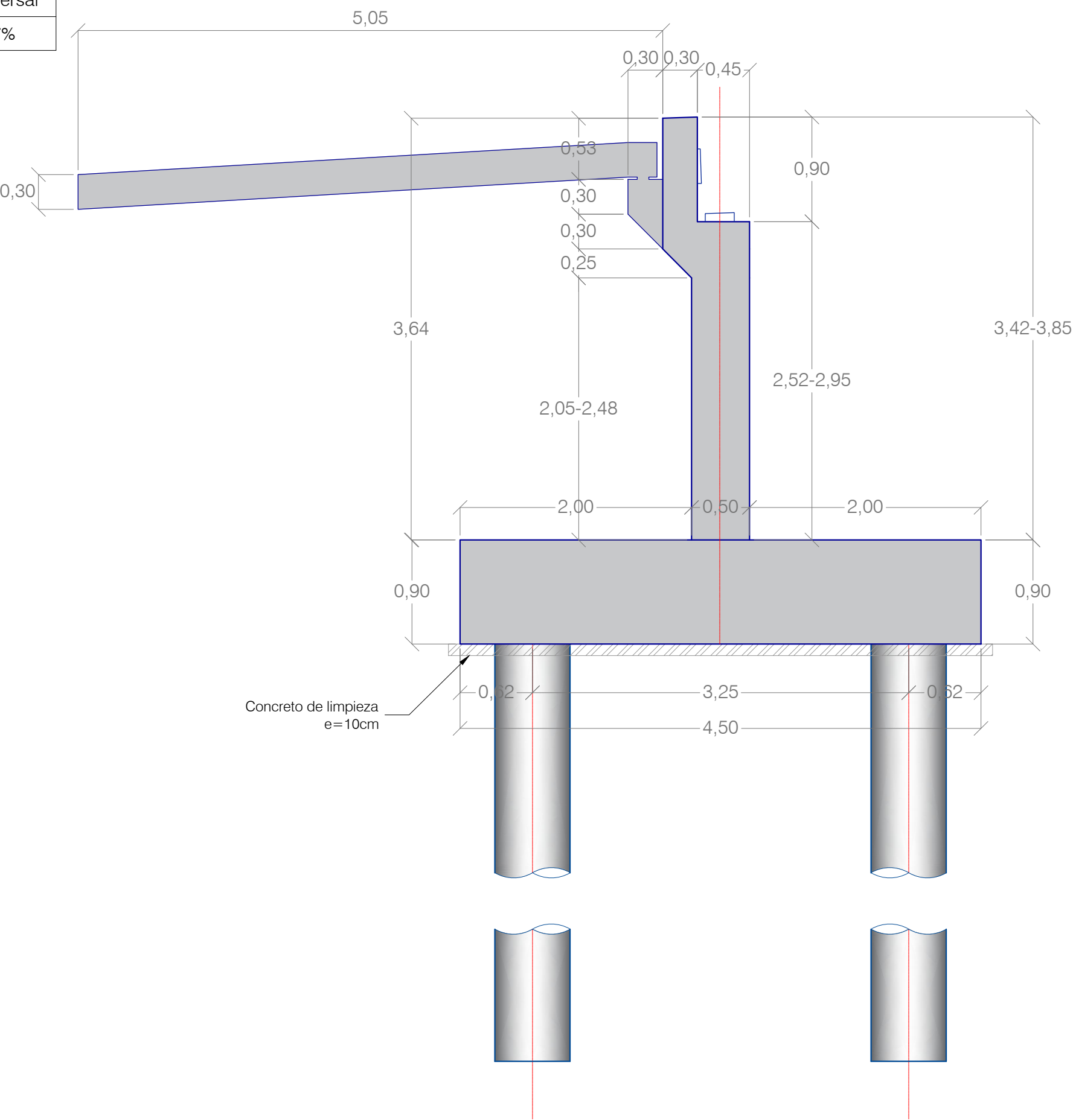
ESTRIBO 1 PERFIL
