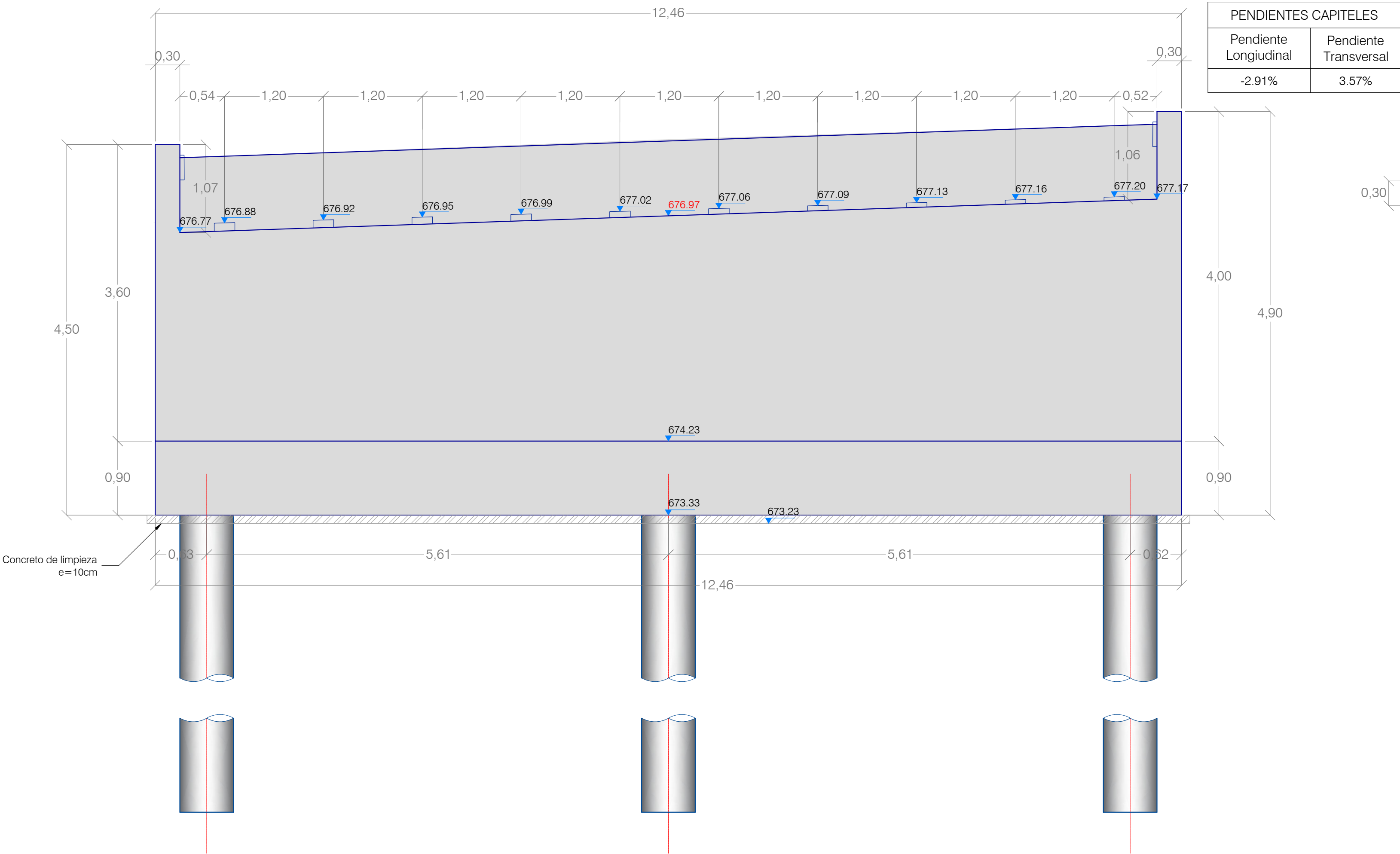
ESTRIBO 1 ALZADO
